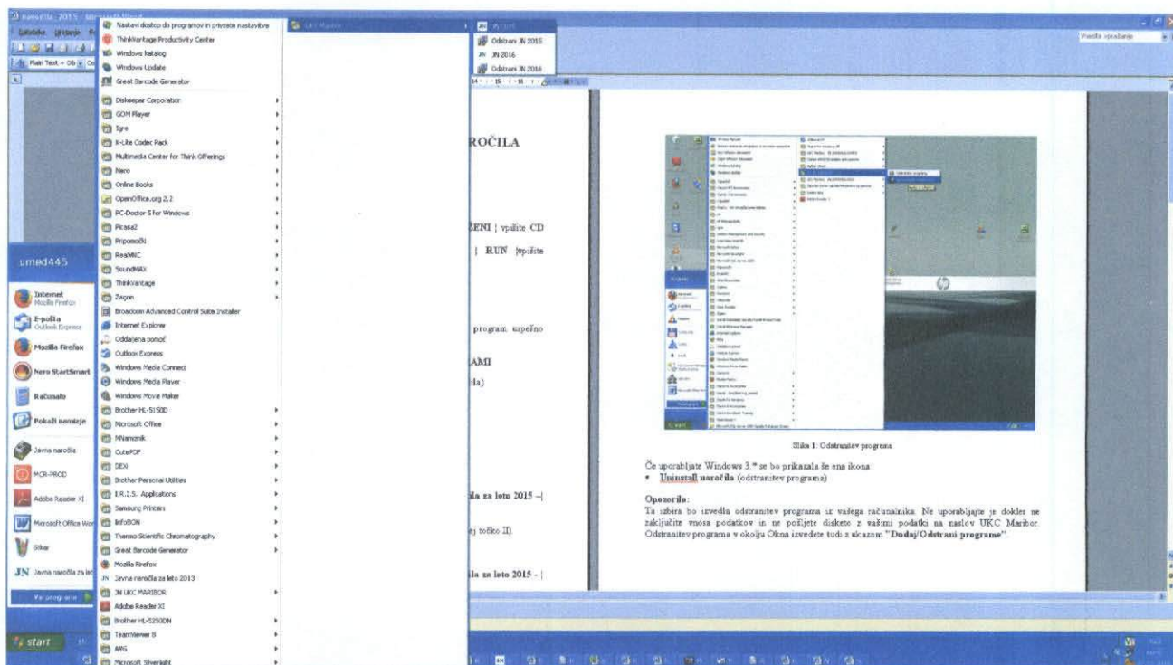
Slika 1: Odstranitev programa
